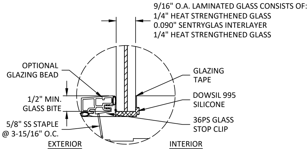
GLAZING DETAIL G2
